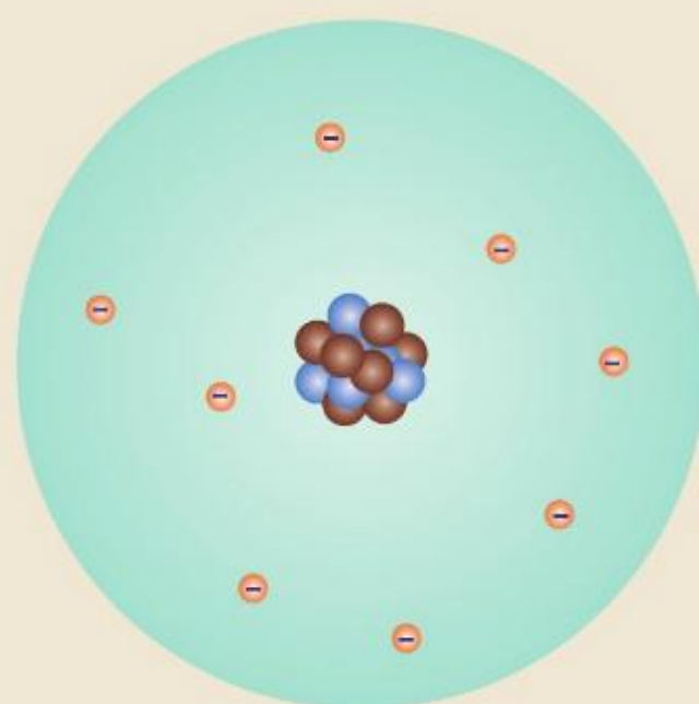
原子内部结构示意图
