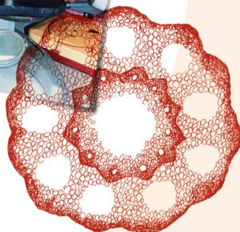
在显微镜下见到的植物茎的剖面
