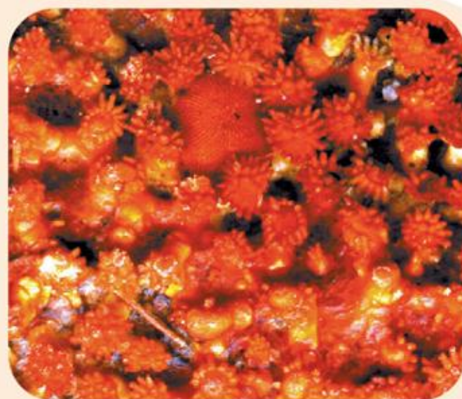
海星局部的放大
