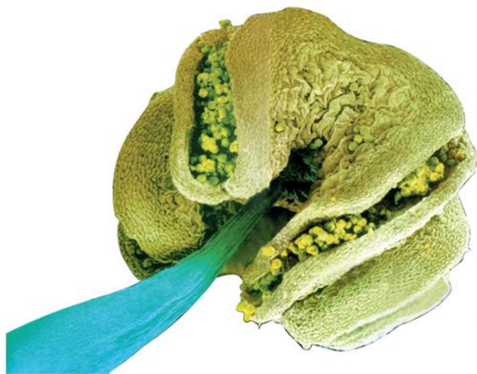
在显微镜下观察到的花粉
